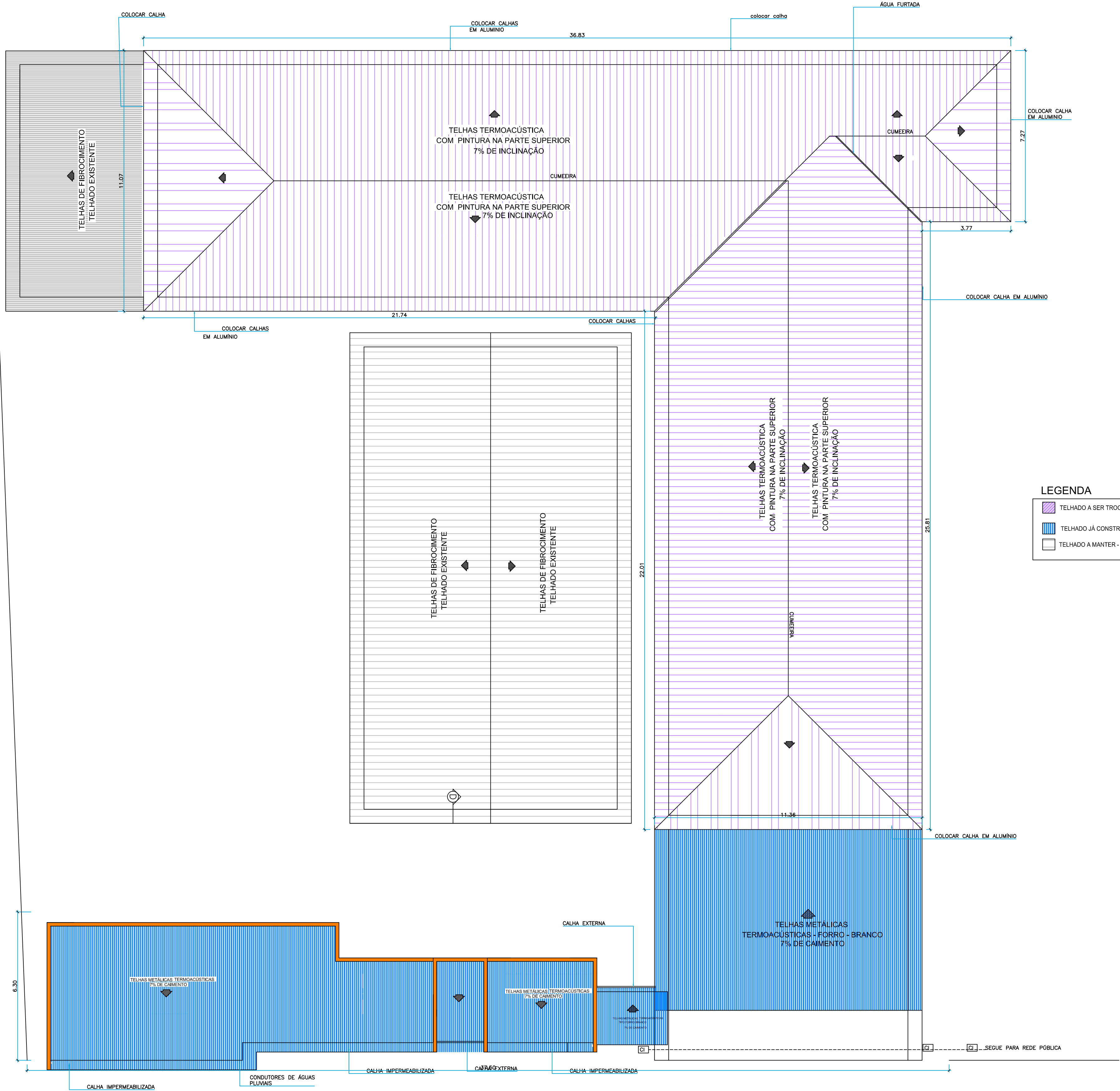
DIAG. COBERTURA ESC.: 1/100
